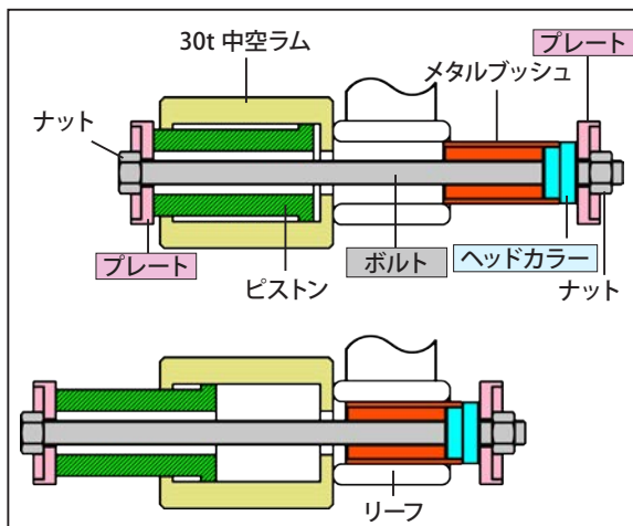
シャックルピン挿入作業 (一例)
