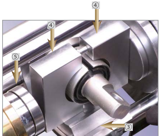
2, 受け金③上に、新品ブッシュを挟んだブッシュコンプレッサー④を、写真のような向きでセットします。この時ブッシュは、できるだけセンターに、また、割れの部分をツールの割れ部に合わせてください。(ブッシュの傷つき防止のため) 本体には当て金⑤をセットし、油圧ポンプを作動させて、ブッシュを圧縮します。
