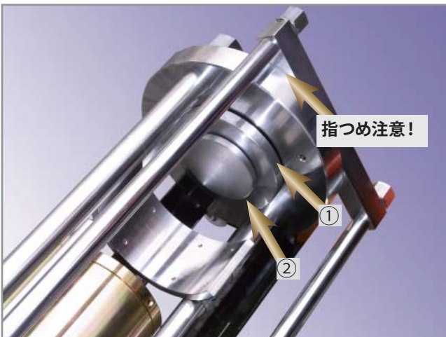
1, フロントプレートに、ガイド①、当て金(大) ②をセットします。
